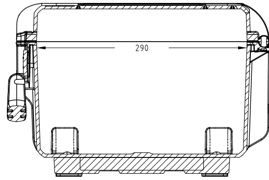
Sezione B-B Section B-B
