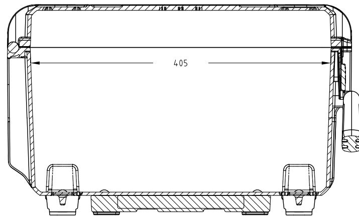
Sezione B-B
