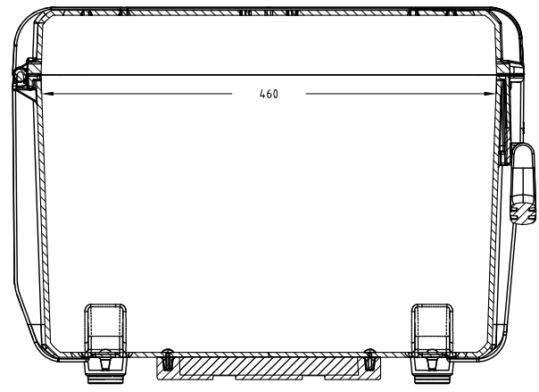
Sezione B-B Section B-B
