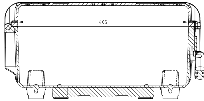
Sezione B-B Section B-B
