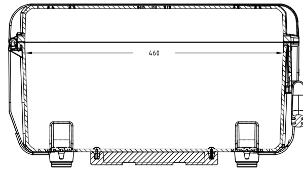
Sezione B-B Section B-B
