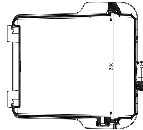
Sezione B-B Section B-B
