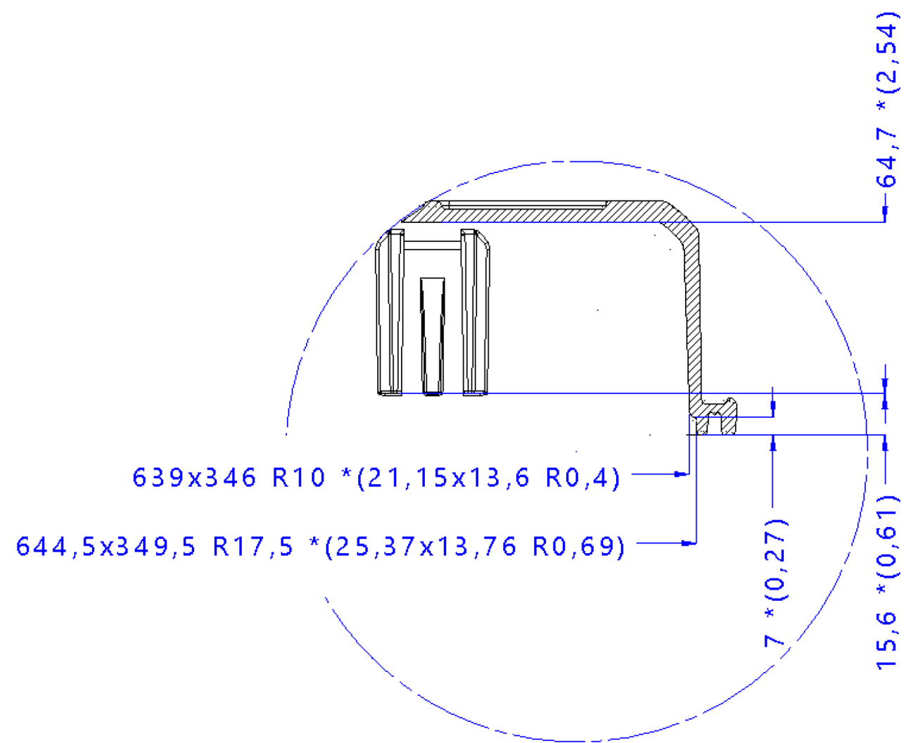
Dettaglio Chiusura Ermetica Coperchio Lid Airtight Closure Detail
